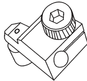
Roller diameter: 4mm 4mm直徑滾輪傍位
