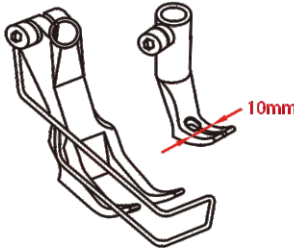
Wider standard feet 加闊標準壓腳
