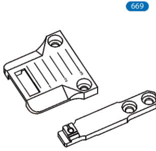
Standard needle plate & feed dog 標準針板及送布牙
