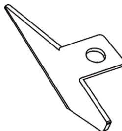
(Improved version of 0667-245004) (0667-245004 改良款式) Center guide 中分傍位
