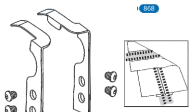
Downturn hemmer attachment 下摺邊助縫配件
