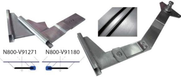
N800-V91271 Left retainer guide + N800-V91180 Right retainer guide N800-V91271 左邊導帶器 + N800-V91180 右邊導帶器
