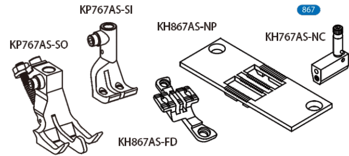
Asymmetric guiding gauge set 不對稱分骨針位
